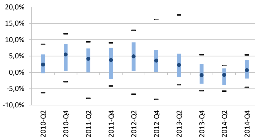
Figura I.9 - Variazioni tendenziali della produzione del mercato danni (premi lordi contabilizzati) Mediana, range interquartilico, 10° e 90° percentile
