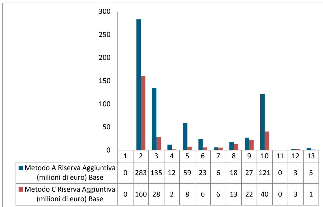
Figura I.36b -Riserve Aggiuntive per rischio di tasso di interesse Appostamento più e meno prudente a raffronto (Metodi A e C)
